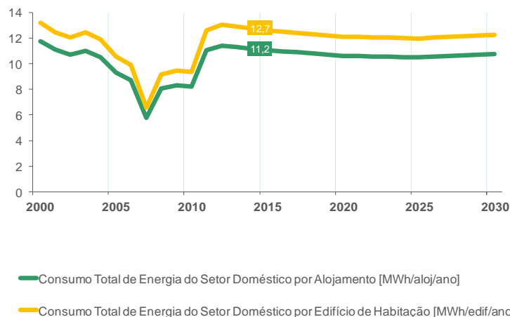
Figura 34 - Consumo Total de Energia do Setor Doméstico por Edifício de Habitação e por Alojamento [MWh/aloj/ano] [MWh/edif/ano]
