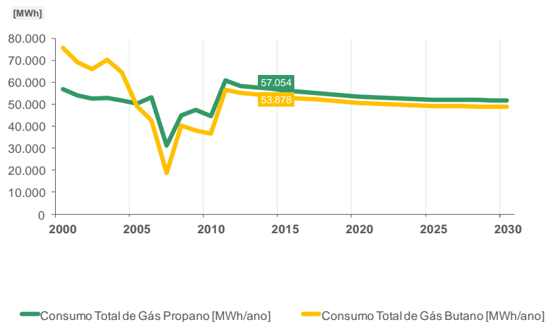
Consumo Total de Gás Butano e de Gás Propano [MWh/ano]
